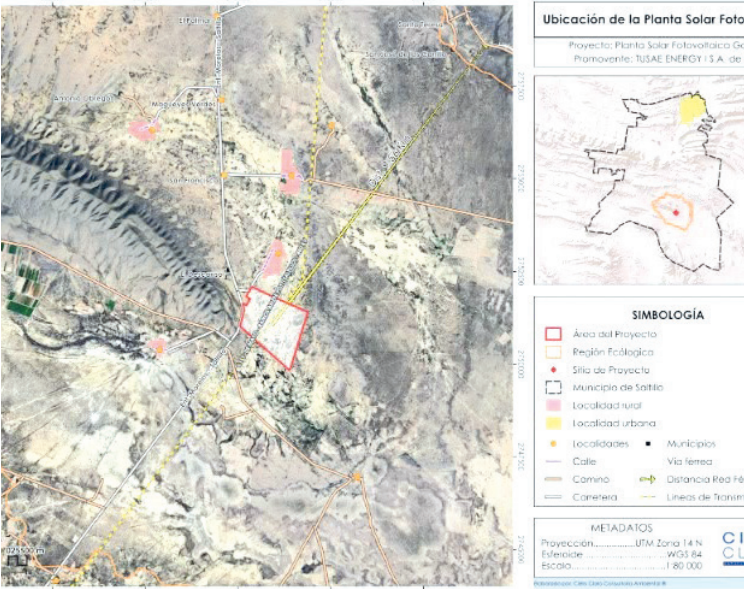
EL PROYECTO CONTEMPLA 172 mil 440 paneles solares, una superficie de 226.47 hectáreas y conexión eléctrica con la red de CFE mediante infraestructura especializada proyectada.
